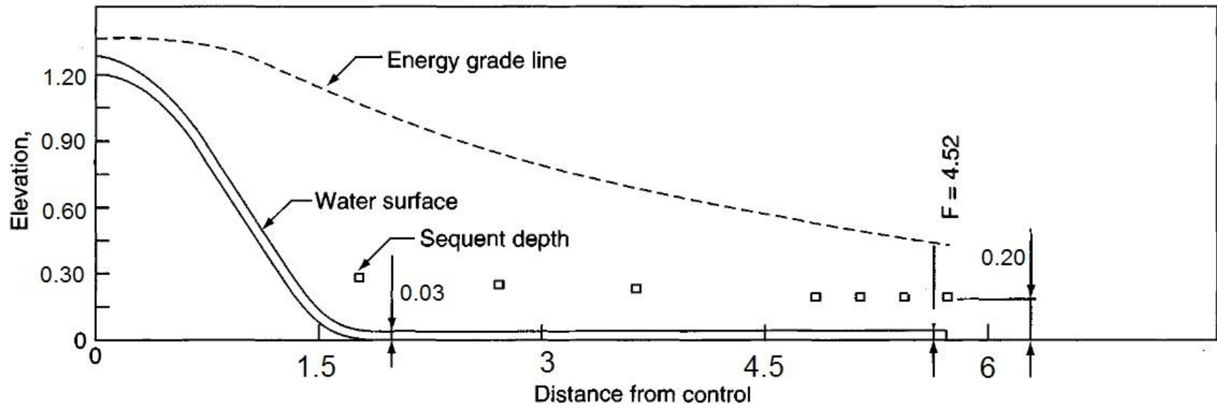
شکل ۴ نیمرخ هیدرولیکی حوضچه ترانشه ای طراحی شده ایستگاه فاضلاب طرح جامع شهر اهواز
