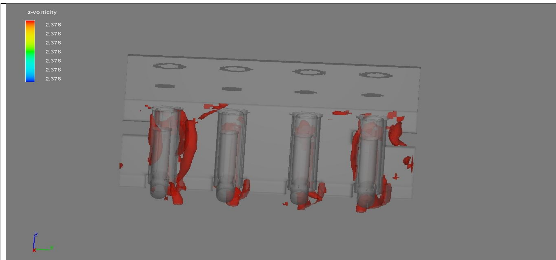
شکل ۲- مدل سازی گردابیهای سطحی و زیر سطحی در حوضچه مکش ترانشه ای با کمک مدل ۳D Folw برای دستیابی به بهترین ابعاد
