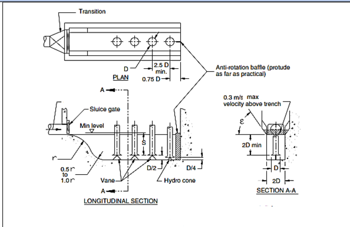
شکل ۱ پلان و مقطع حوضچه مکش طراحی شده مطابق توصیه استاندارد ۹,۸۵ ANSI/HI
