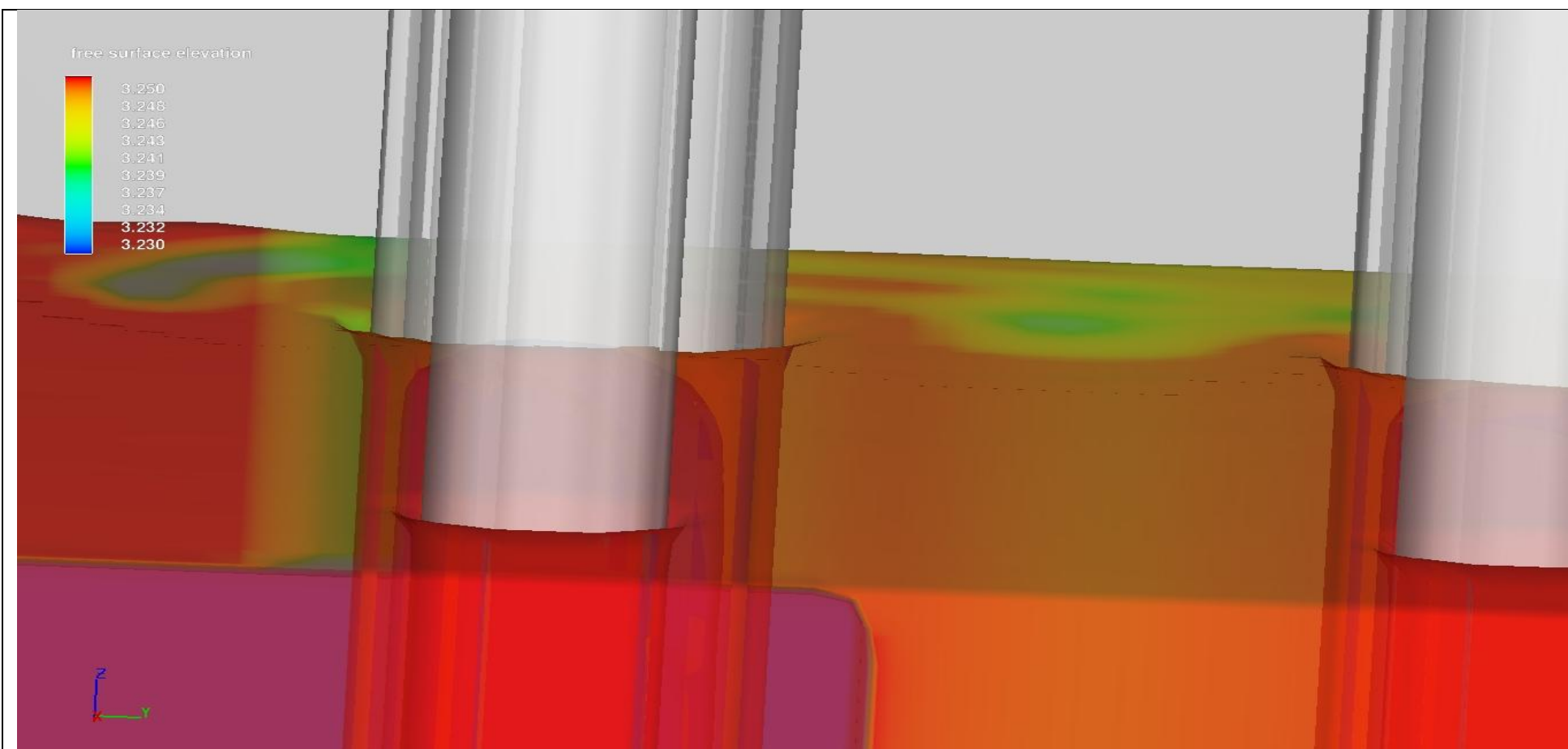
شکل ۳- تغییرات تراز آب در اثر شکل گیری گردابه‌های سطحی در مدل ۳D Flow
